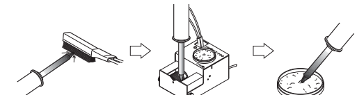
(1) ストレートブラシで酸化物 (2) ハッコー FT-700 で (3) ハッコー FS-100 で を除去します。 再度クリーニングし 再はんだめっきし ます。 ます。
