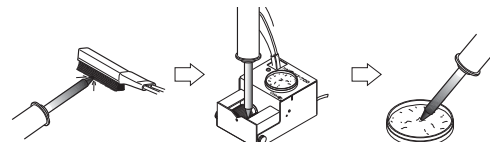
(1) 用刷子除去氧化物。 (2) 用HAKKO FT-700再次清潔。 (3) 用HAKKO FS-100再次搪錫。
